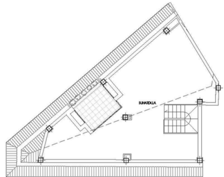
Planta Bajo Cubierta
