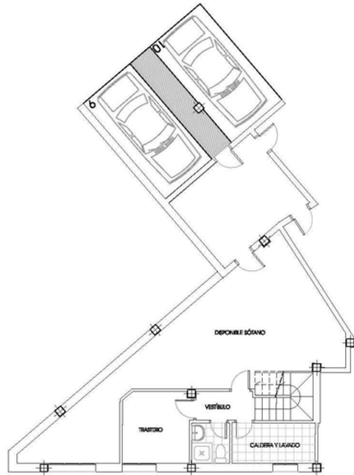
Planta Sótano
